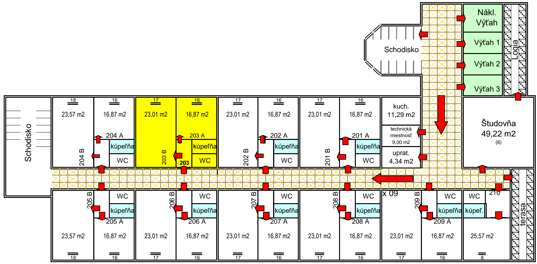
Školský internát 2.poschodie
